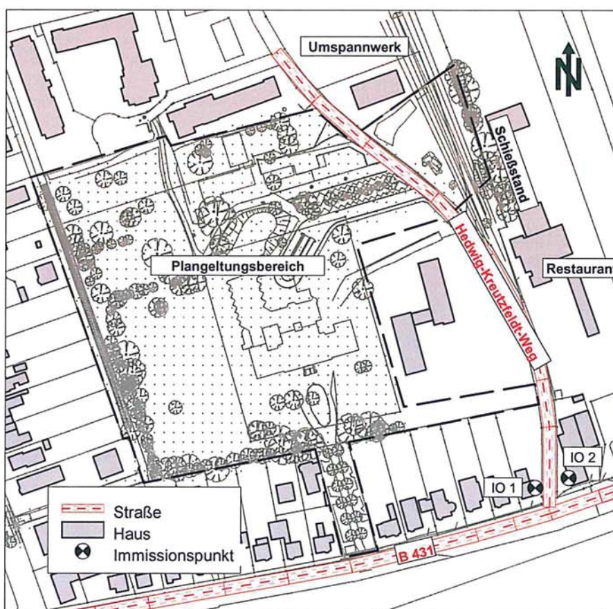
Abb. 17 Lageplan mit Darstellung der Lärmquellen (lt. Gutachten vom 16.04.2013)
